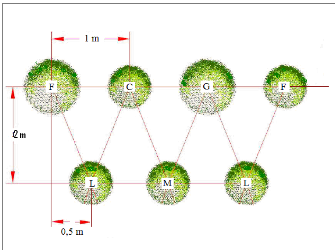
Figura n. 71: schema realizzazione impianto essenze arbustive
