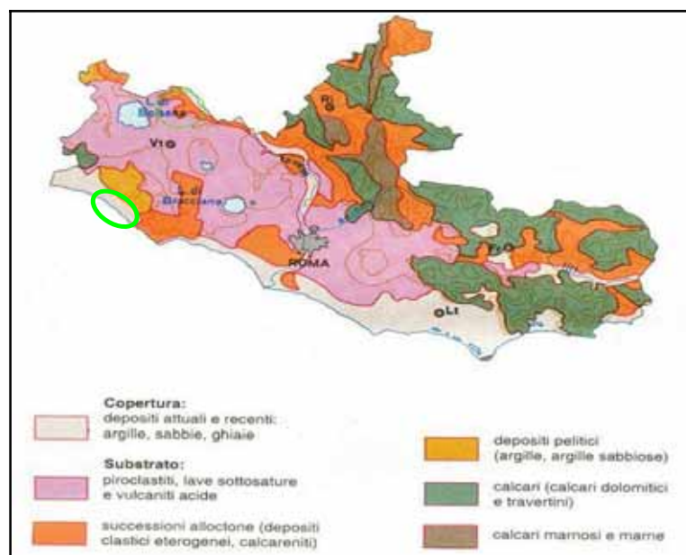
Figura n. 20: carta litologica del Lazio (in verde il comprensorio in esame)
