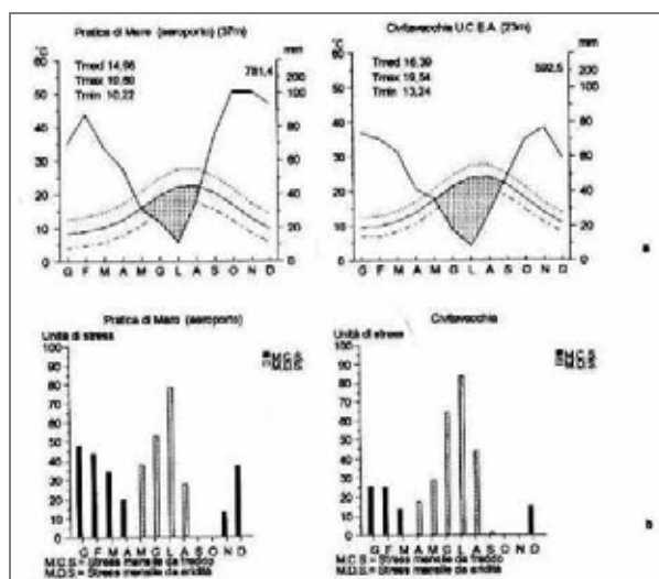
Figura n. 18: diagrammi Bagnouls-Gaussen (a) e Mitrakos (b) delle stazioni pluviometriche relative all'unità fitoclimatica 13 (da Carta del Fitoclima del Lazio, Assessorato Agricoltura e Foreste, Caccia e Pesca della Regione Lazio, 1994 )
