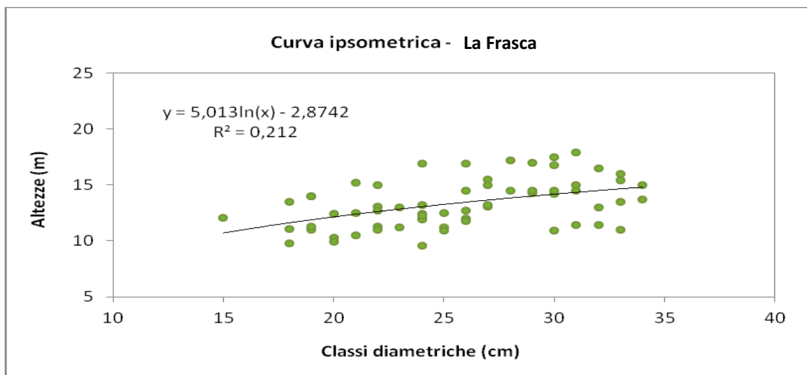
Figura n. 53: curva ipsometrica – La Frasca
